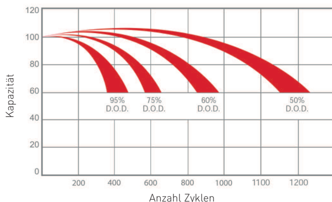
Ladezyklen (25°C)
